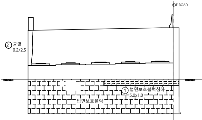
정면도
